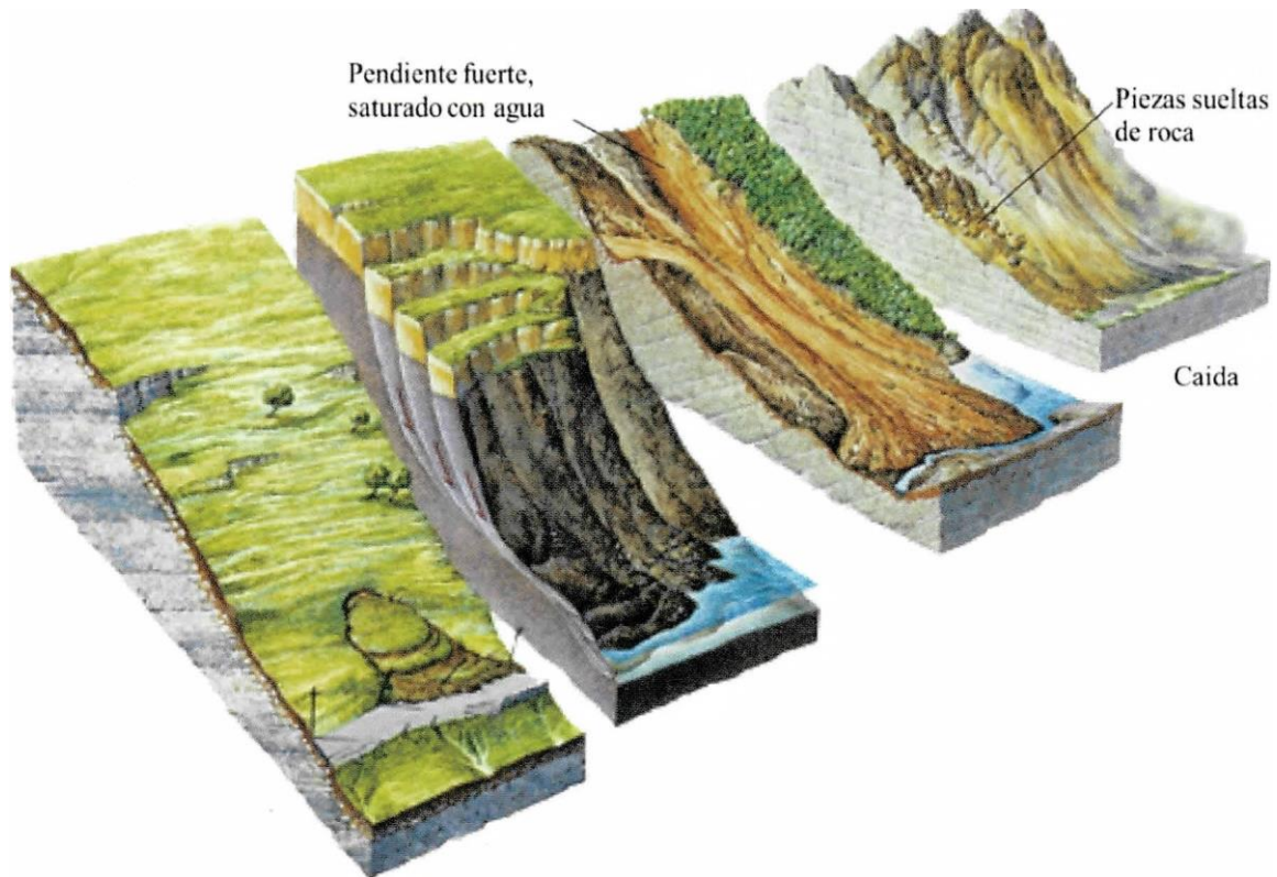
Figura N°3. Tipos de deslizamientos con la formación geomorfológica de la Tierra.
