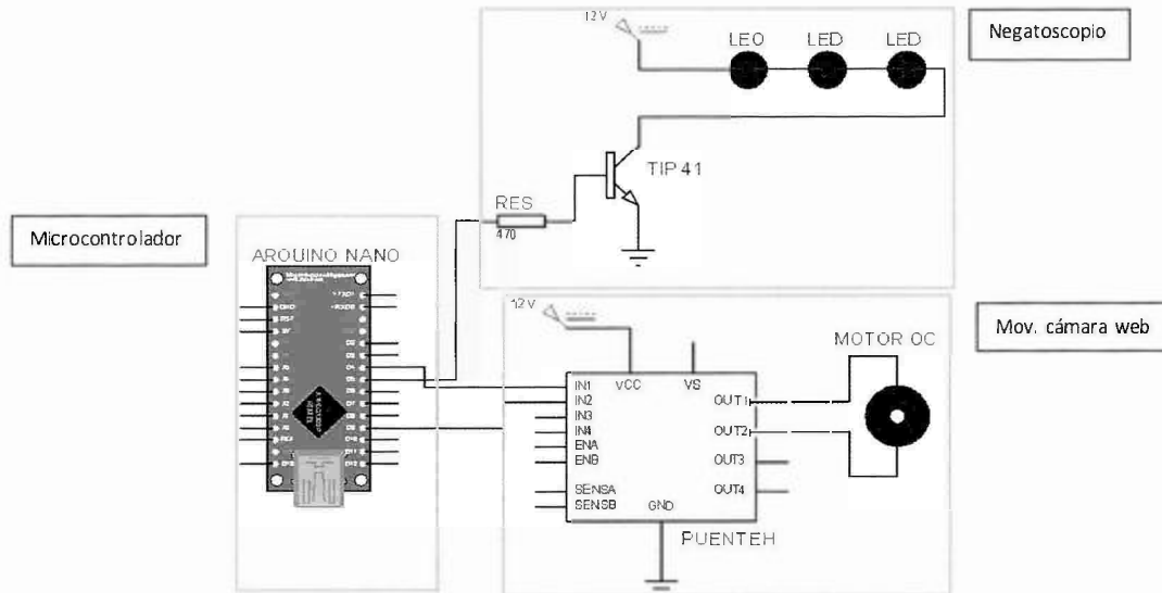
Figura N°1. Esquema del circuito electrónico del Hardware
