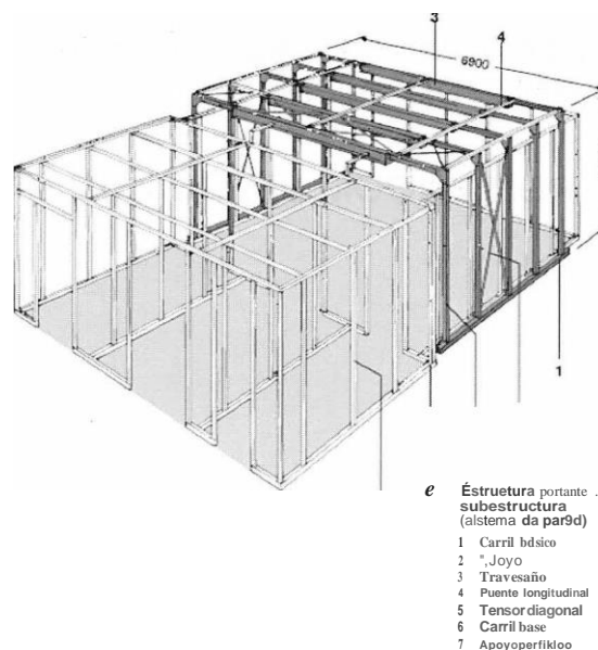
Figura N° 1. Subestructura metálica portante
