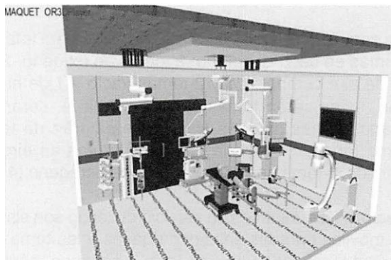
Figura N° 4. Diseño sala de cirugía tipo A "equipada"
