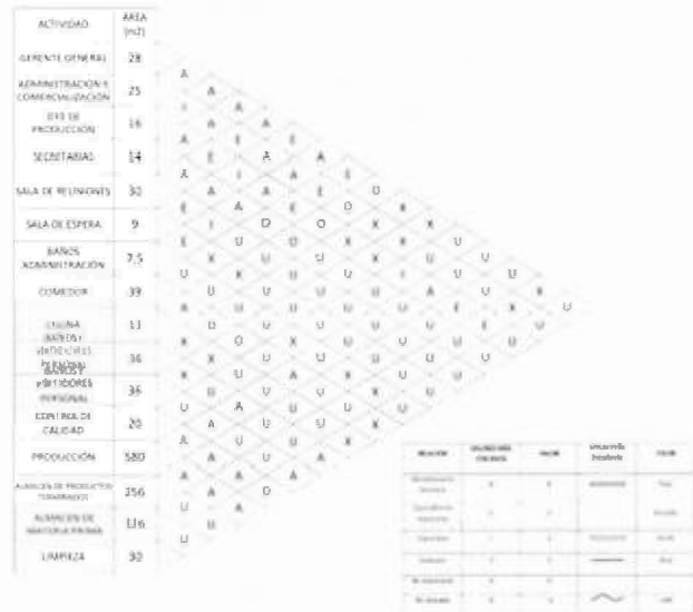
Diagrama N° 1. Relaciones de la Planta Procesadora de Harina de Yuca
