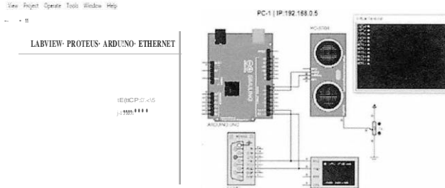
Figura Nº 12. Envío y recepción de datos virtuales a través de Ethernet
