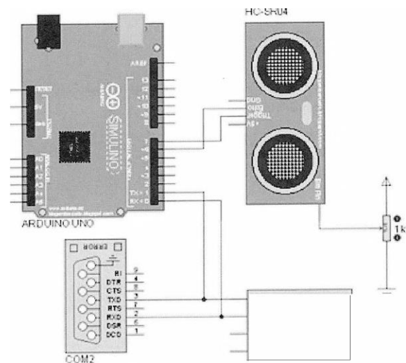
Figura N° 1. Circuito para la medición de distancia
