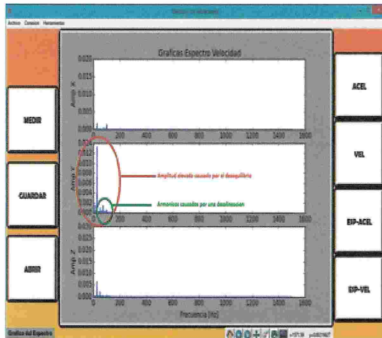
Figura N° 7. Espectro de vibración medido del banco de pruebas
