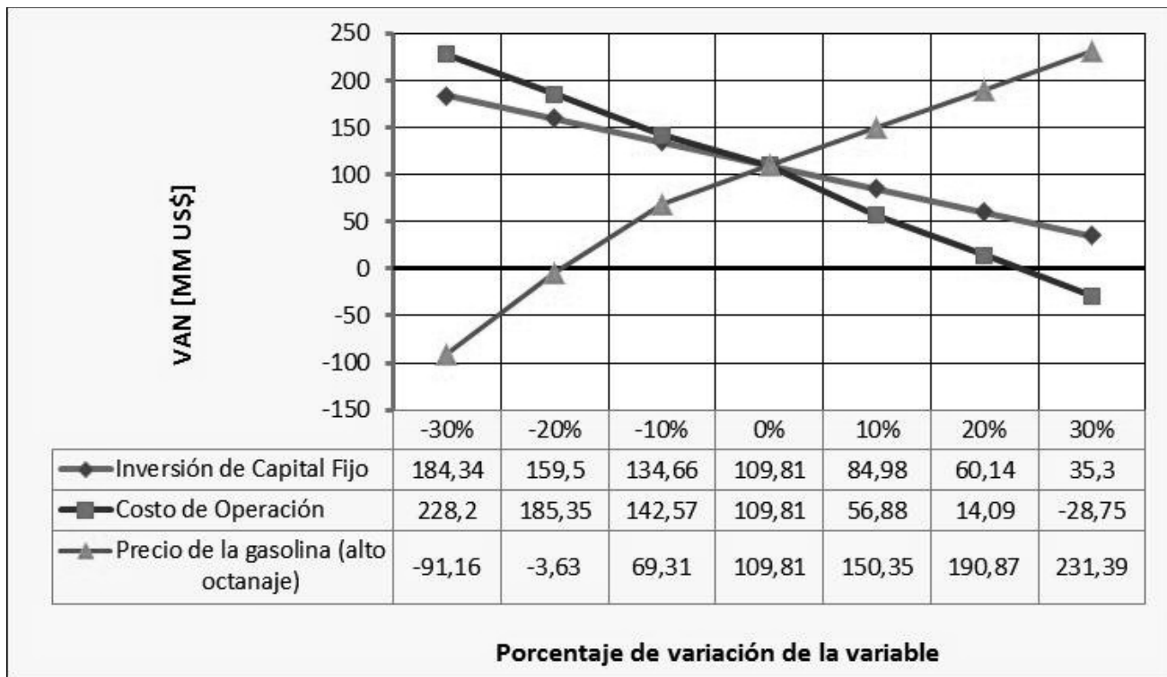
Figura N° 16. Análisis de sensibilidad
