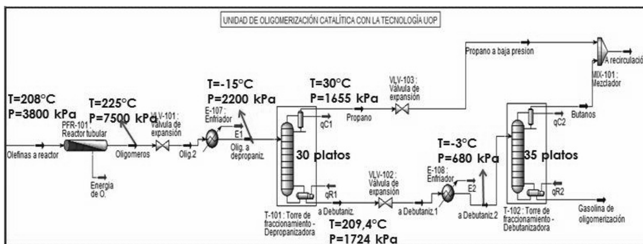
Figura N° 13. Simulación de la Unidad de Oligomerización Catalítica
