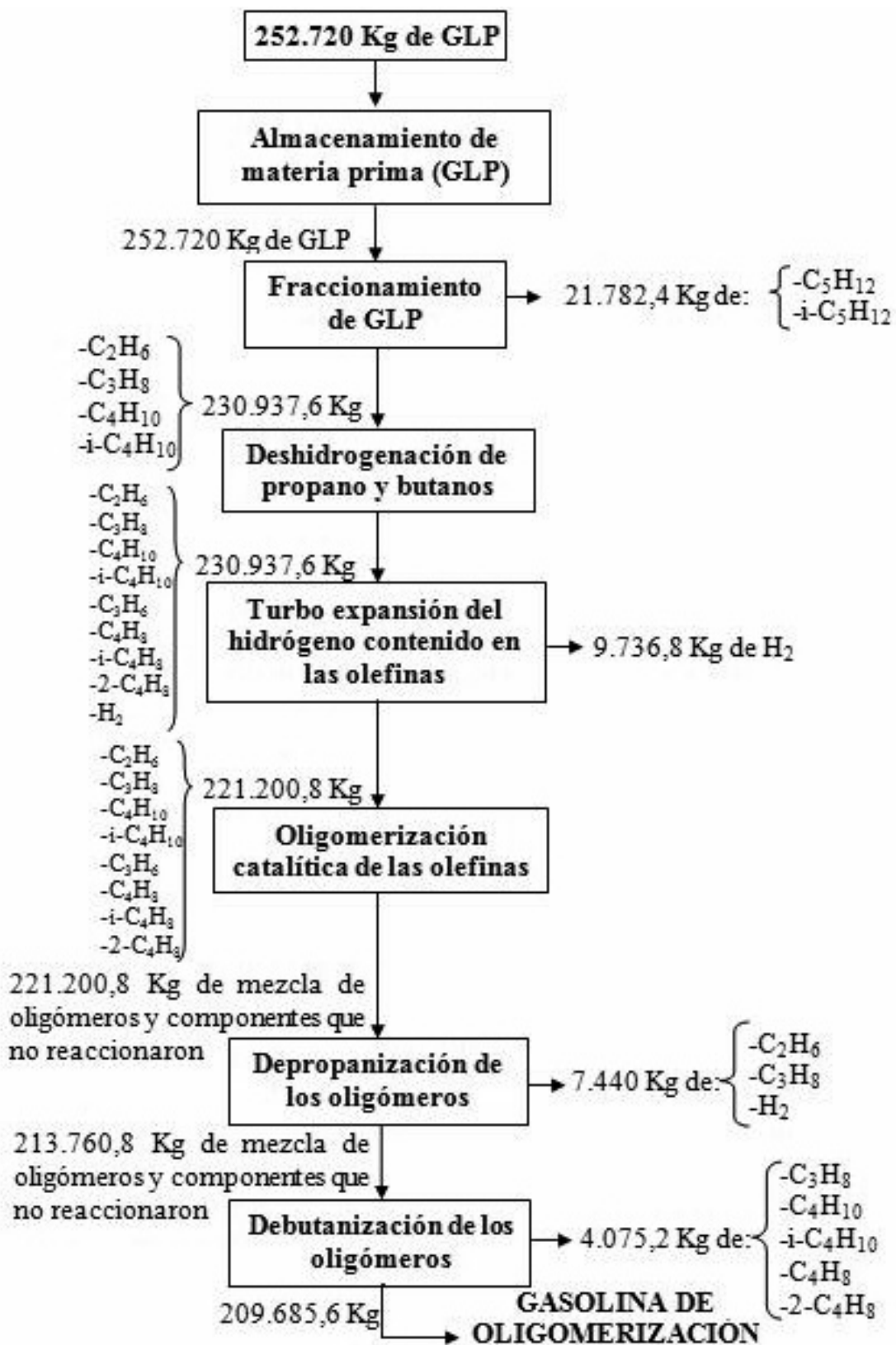
Figura N° 14. Balance de masa de la Planta de Oligomerización Catalítica
