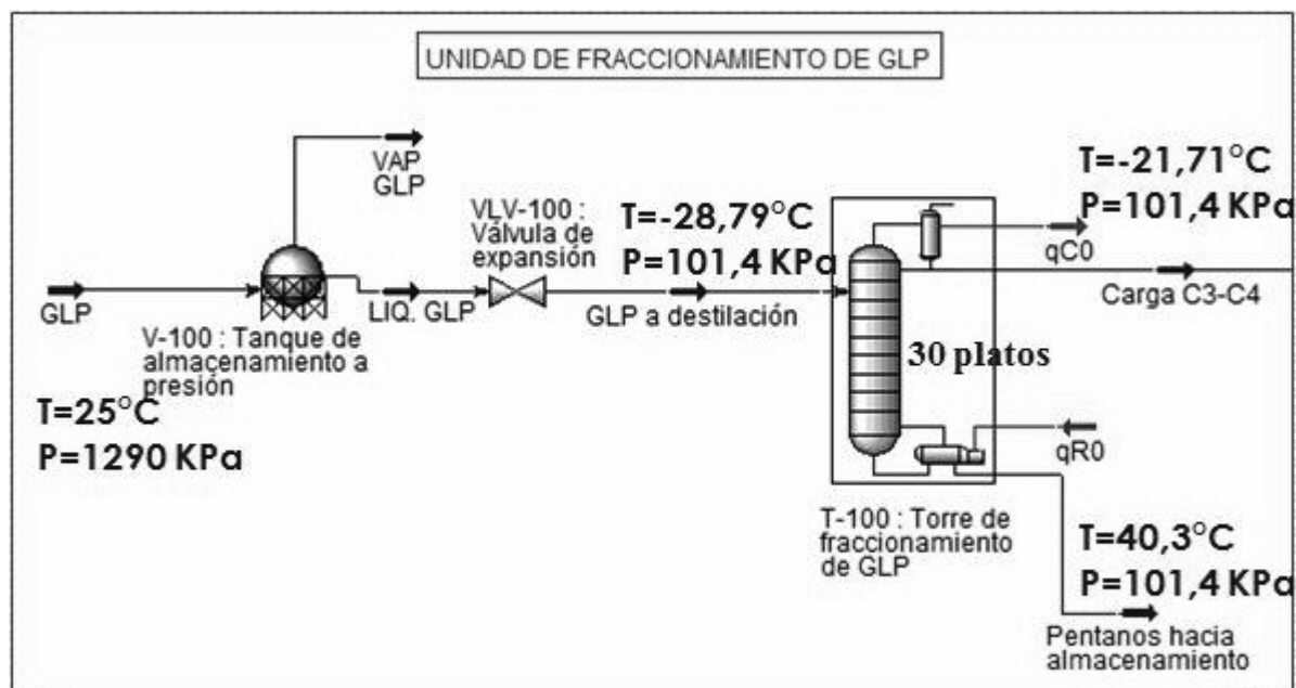
Figura N° 10. Simulación de la Unidad de Fraccionamiento de GLP
