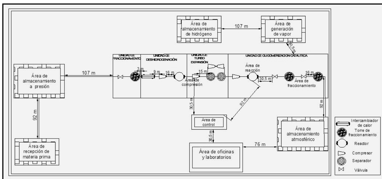
Figura N° 15. Layout de la planta de Oligomerización Catalítica
