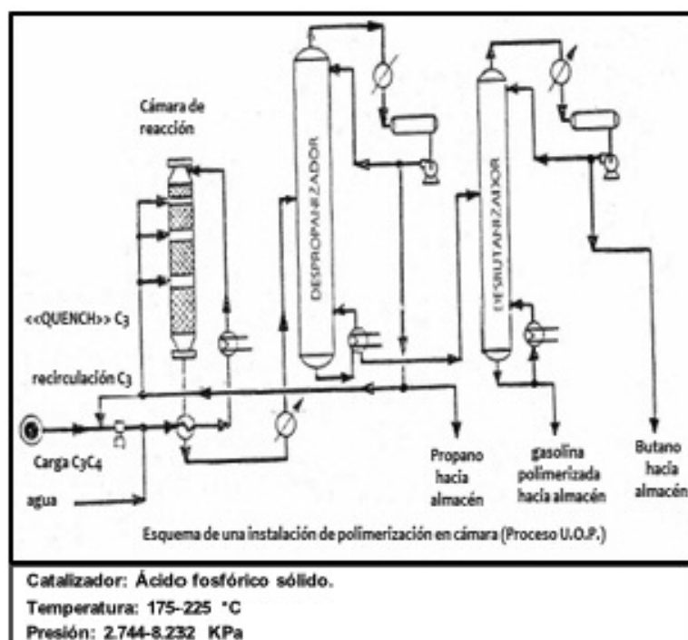
Figura N° 9. Variables de operación y esquema de instalación del Proceso U.O.P
