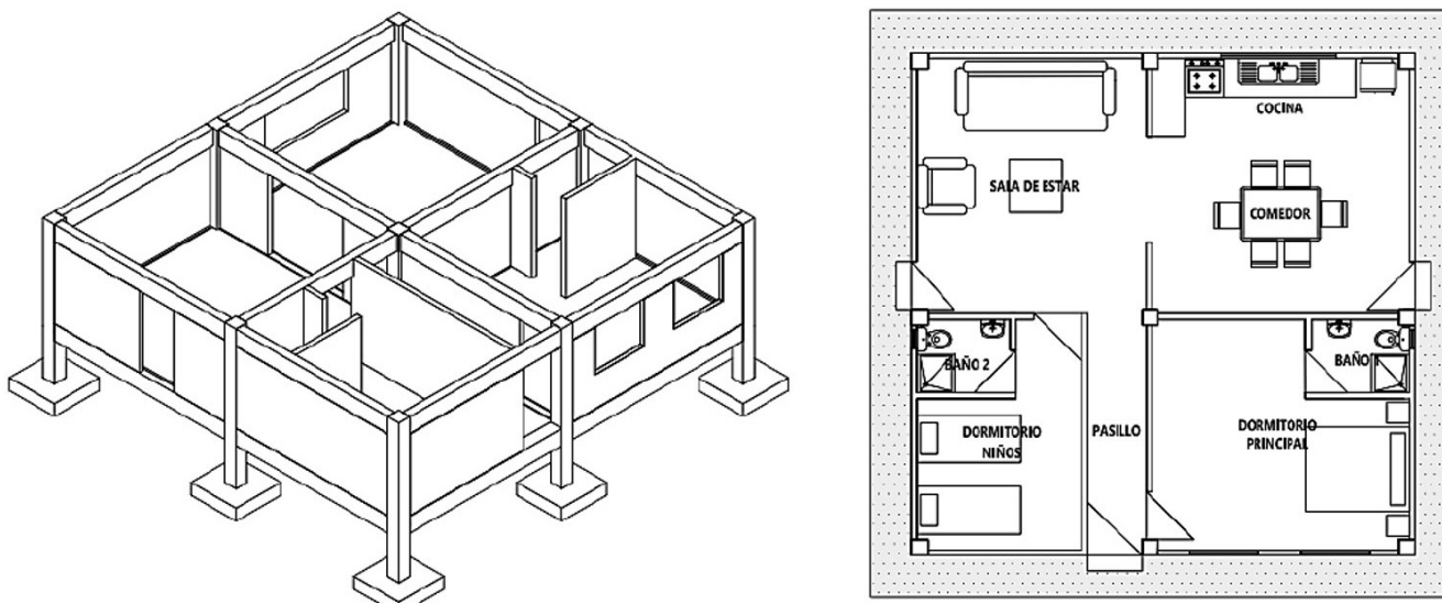
Figura N° 7. Vivienda convencional generada para la comparación de costos
