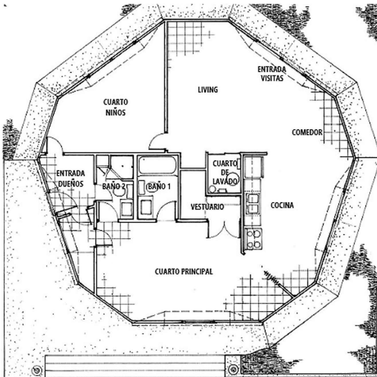
Figura N° 3. Vista en planta del proyecto de vivienda
