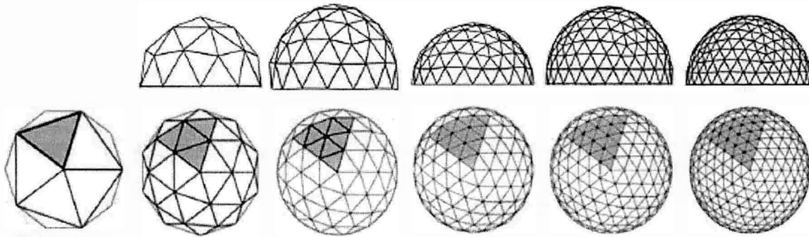
Figura N° 1. Domos geodésicos de R. B. Fuller
