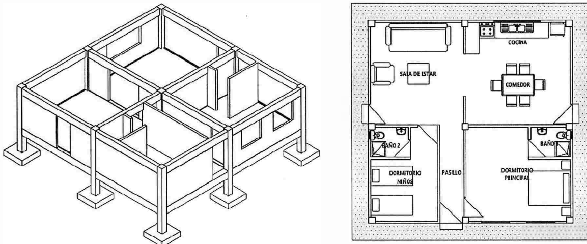
Figura N° 7. Vivienda convencional generada para la comparación de costos
