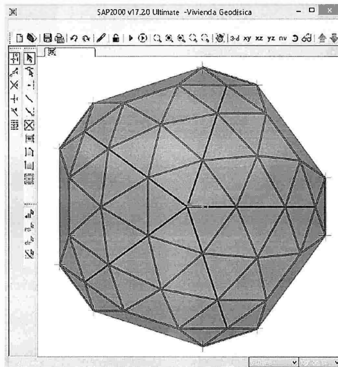
Figura N° 5. Geometría del modelo matemático dentro del programa SAP2000®
