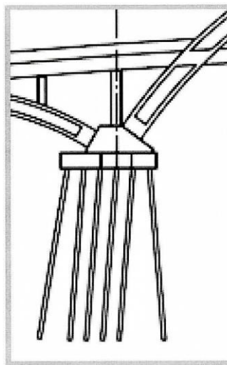
Figura 5 Diseño Final Micropilotes
