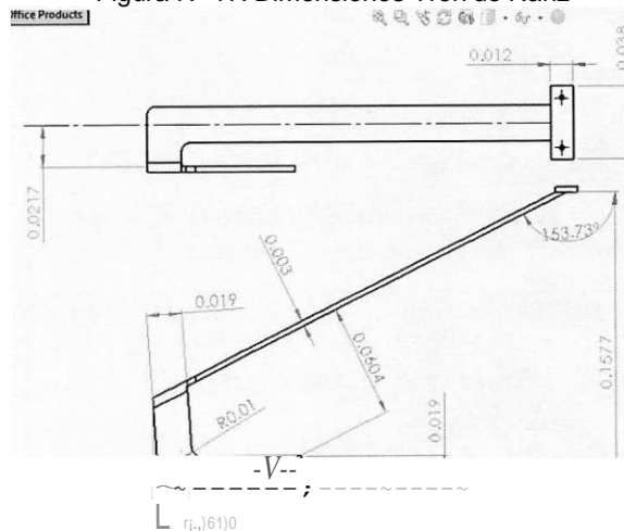
Figura N° 17. Dimensiones Tren de Nariz
