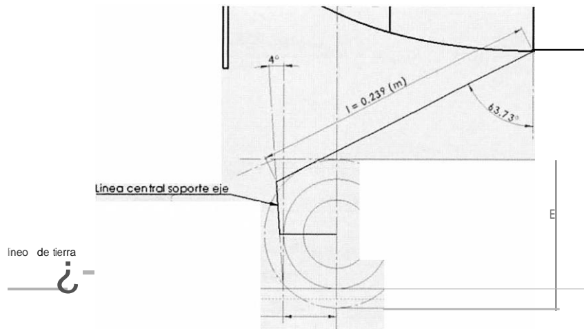
Figura N° 9. Geometría del Tren de Nariz
