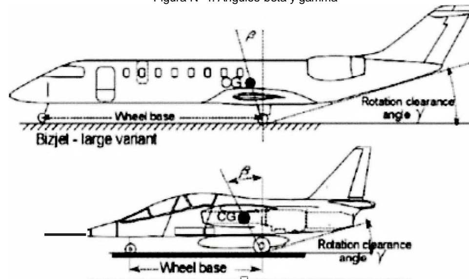
Figura N° 4. Ángulos beta y gamma
