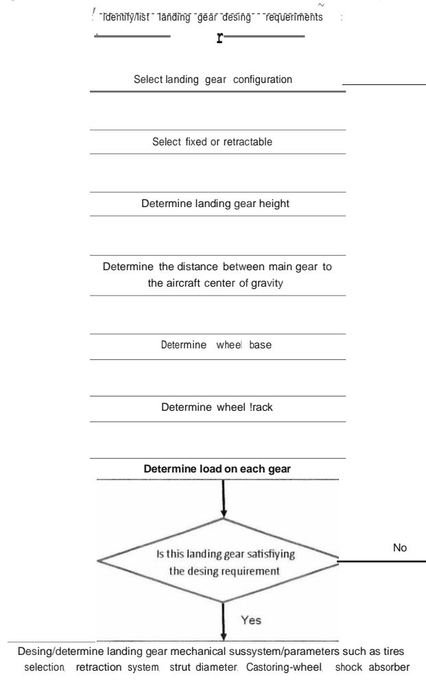
Figura N° 2. Pasos para el diseño de Tren de Aterrizaje
