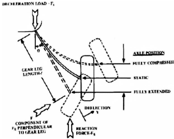
Figura N° 5. Variables de un Tren tipo Cantilever
