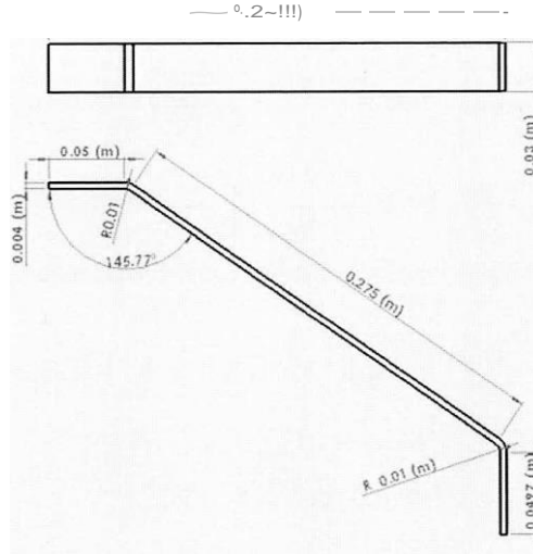
Figura N° 16. Dimensiones Tren Principal
