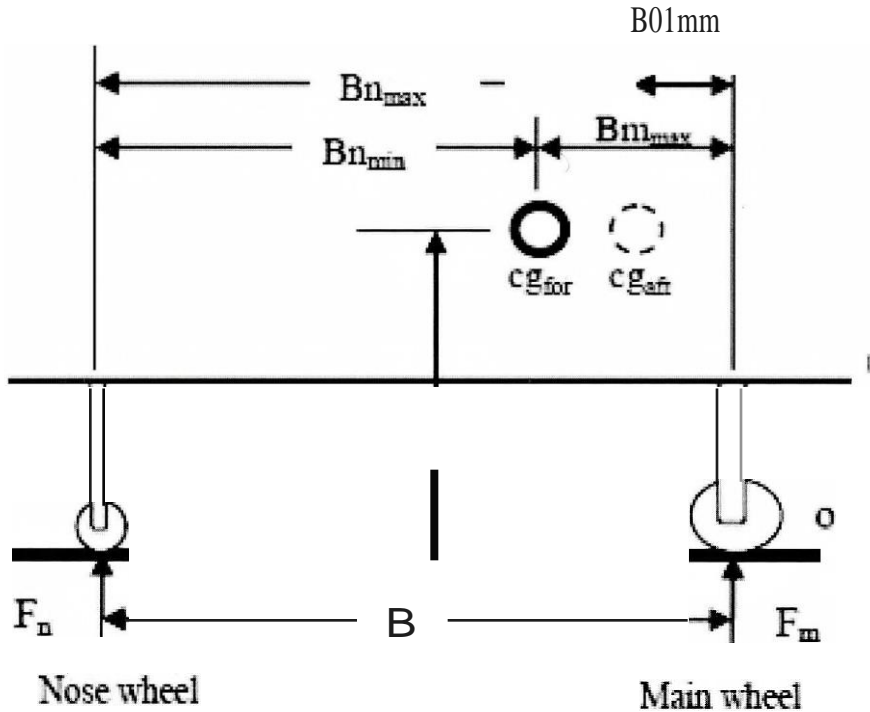
Figura N° 3. Distribución de cargas en trenes de aterrizaje
