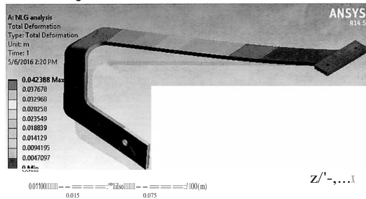
Figura N° 19. Resultados de deformación total
