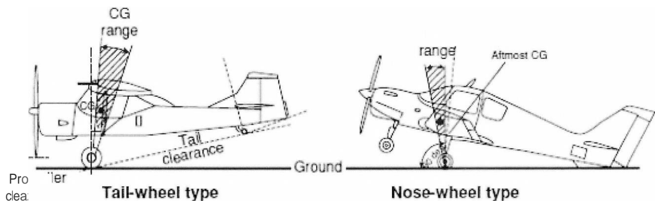
Figura N° I. Tipos de Tren de Aterrizaje más comunes
